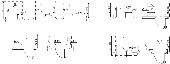
圖205.2.4.2 推開門之操作空間
