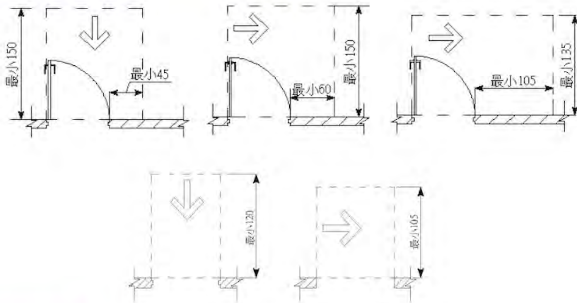
圖304.2.4.3 無門扇之開口所需之操作空間
