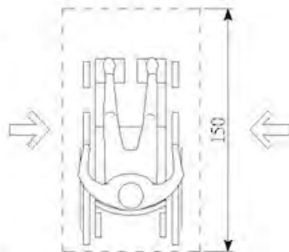
由左右側進入 圖703.2.2
